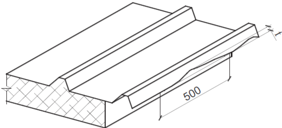
Рисунок 17 - Схема измерения отклонения кромки свободного гофра стыка
