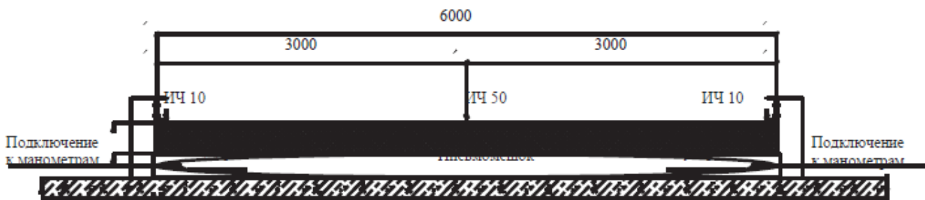
Рисунок Б.6 - Схема испытательной установки
