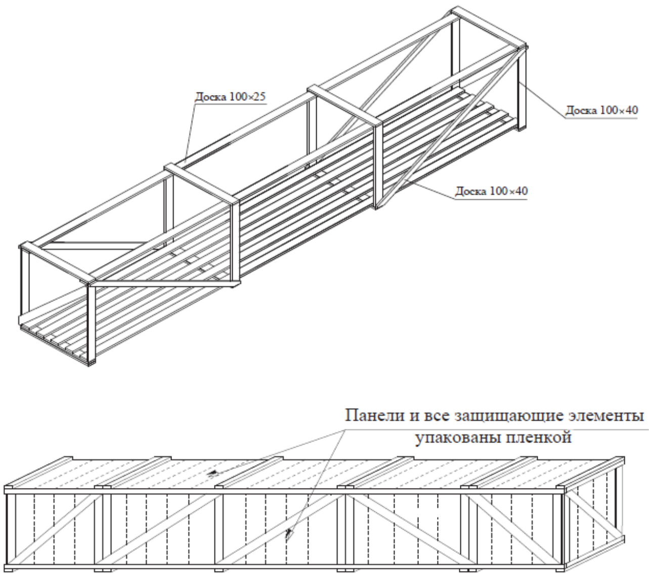
Рисунок А.3 – Пример деревянного контейнера решетчатого типа
