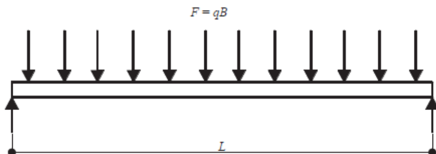
Рисунок Б.3 - Воздействие воздушного давления или вакуума
