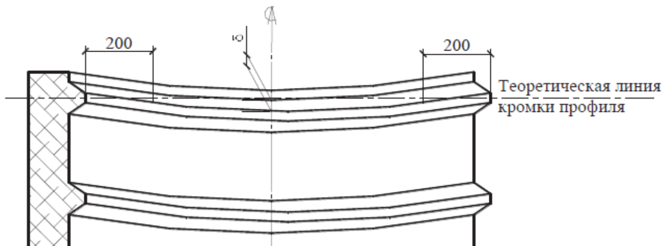
Рисунок 13 - Схема измерения серповидности
