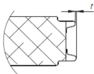
Рисунок 15 - Схема измерения смещения продольных кромок
