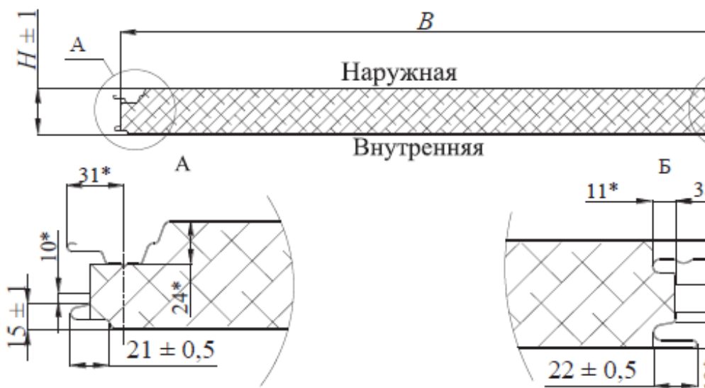
Рисунок 3 - Стеновая панель с симметричным замком по толщине панели, который образует стык в шпунт - открытое крепление (Z)
