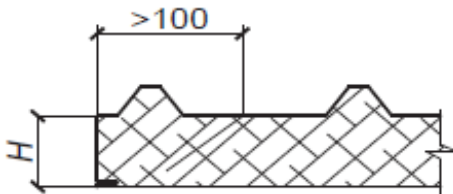
Рисунок 10 - Схема измерения толщины панели
