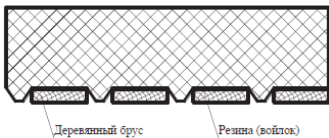
Рисунок Б. 5 - Схема деревянных прокладок
