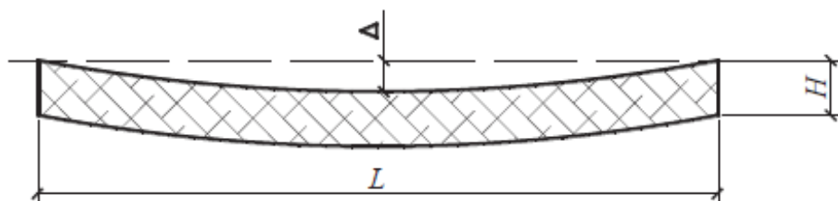
Рисунок 14 - Схема измерения прогиба панели
