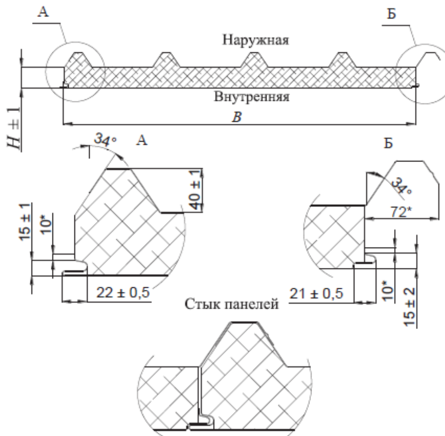
Рисунок 1 - Виды профилирования поверхности металлических облицовок
