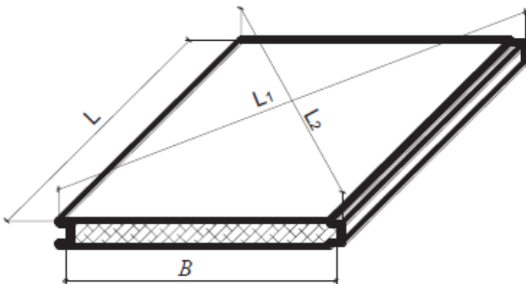
Рисунок 11 - Схема измерения косины реза панели
