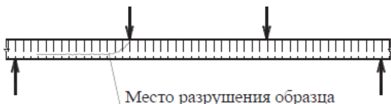
Рисунок В.5 - Типичная схема разрушения сердцевины от сдвига
