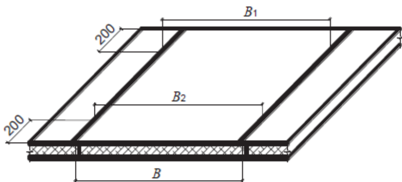
а) Схема измерения рабочей ширины кровельной панели
