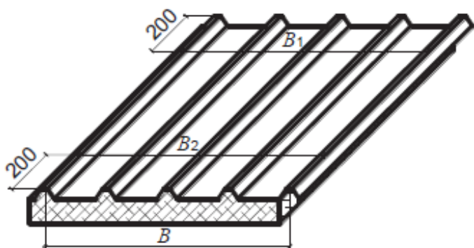
а) Схема измерения рабочей ширины кровельной панели
