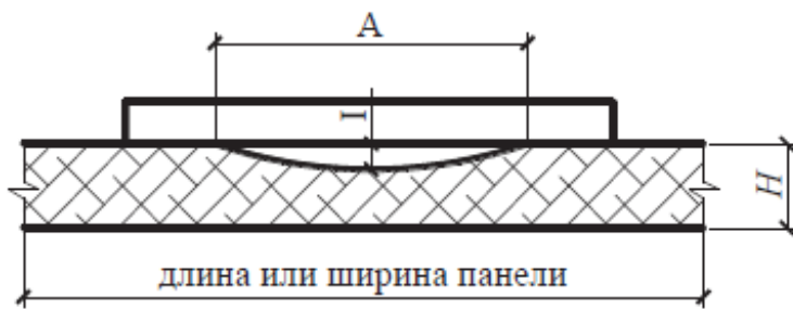
Рисунок 16 - Схема измерения отклонения от плоскостности
